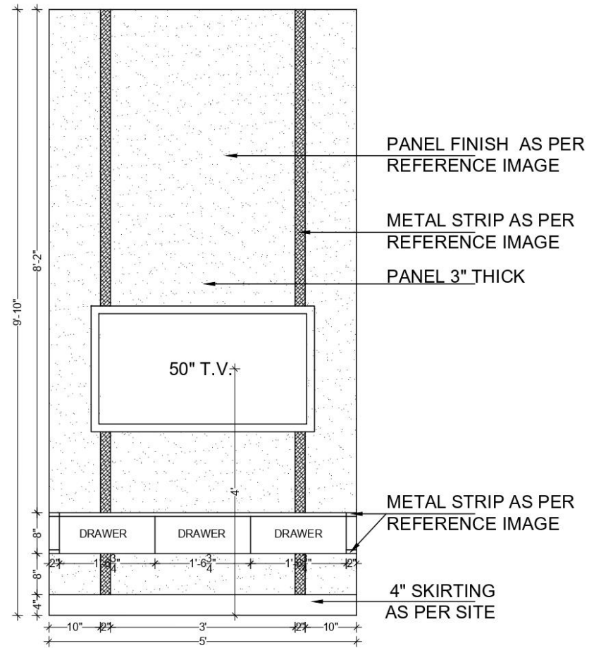
ELEVATION
