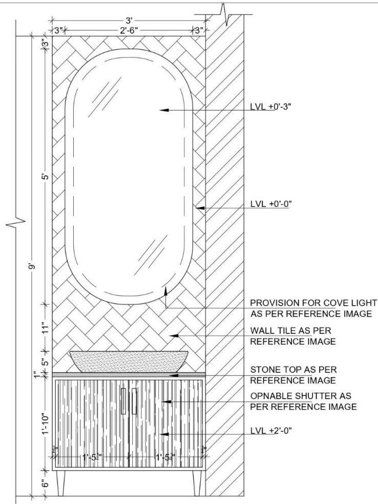
ELEVATION
