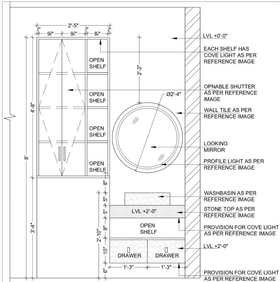
ELEVATION
